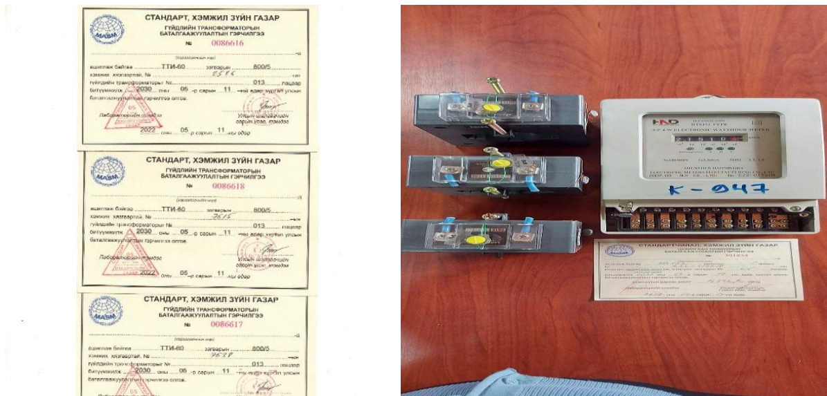
Зураг 5. Цахилгааны тоолуур, гүйдлийн трансформатор
